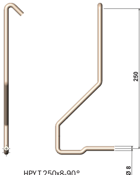
HPYT 250x8-90°
